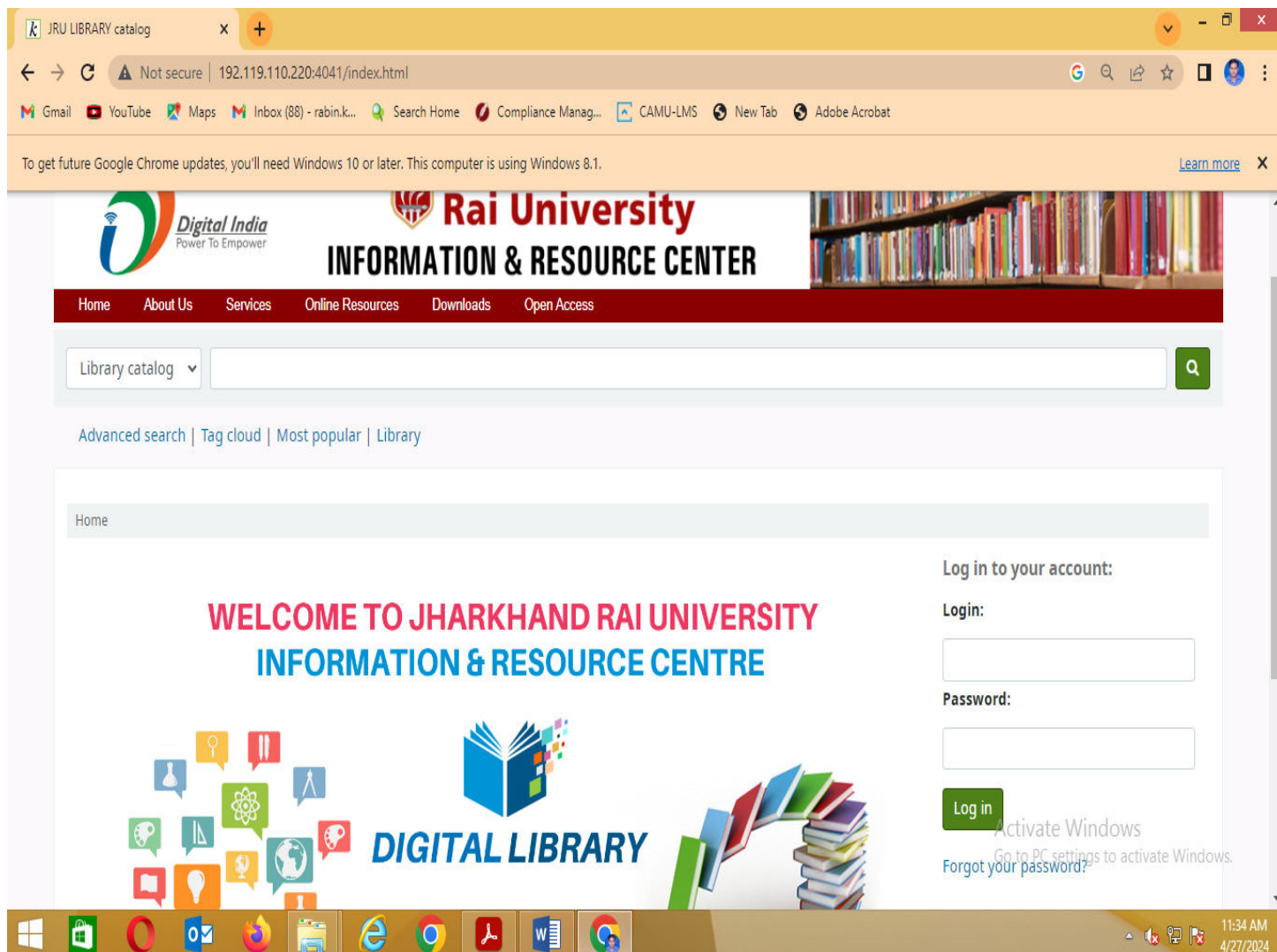
Fig9: WebOPAC
